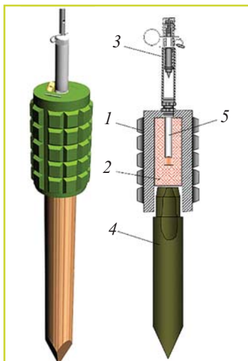
1 – корпус; 2 – взрывчатое вещество – 75 г тротил; 3 – взрыватель; 4 – колышек; 5 – запал
