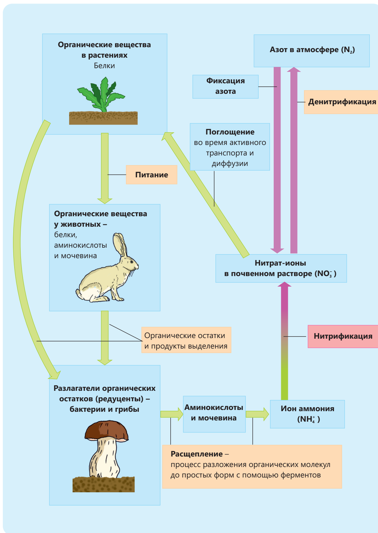
Круговорот азота
