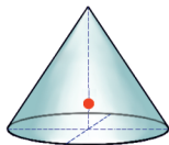
Şəkil 4. Konus, piramida və yarımkürənin ağırlıq mərkəzləri.
