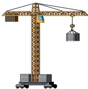
Şəkil 1. Cismə qüvvə təsir edərkən o, yerini dəyişirsə, mexaniki iş görülür.
