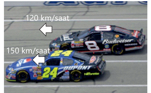
Şəkil 3. Bərabər kütləli avtomobillərdən sürəti böyük olanın kinetik enerjisi daha böyükdür.
