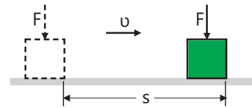
Şəkil 4. Qüvvə iş görmür.
