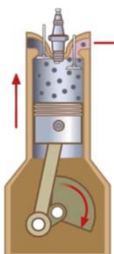
Şəkil 4. Dördtaktlı karbürətorlu mühərrikin iş prinsipi.
