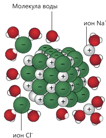
Электролитическая диссоциация хлорида натрия
