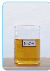
Метилоранж в щелочной среде становится жёлтым.
