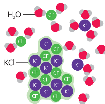
Электролитическая диссоциация хлорида калия
