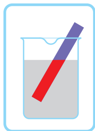
Синяя лакмусовая бумага в кислой среде окрашивается в красный цвет.
