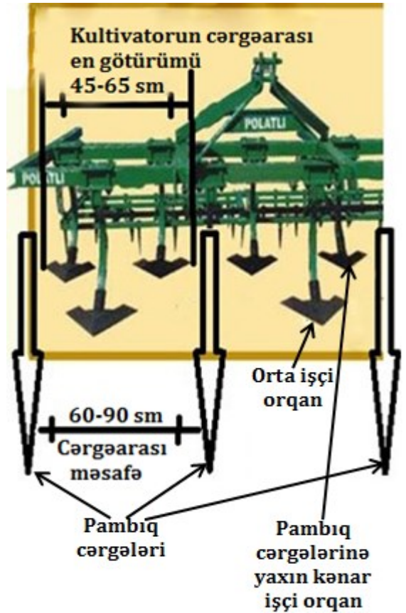
Şəkil 4.8. Pambığın cərgəalarını becərən kultivatorun iş sxemi
