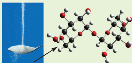
Строение сахара
