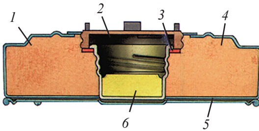
TM-62M ნაღმის აგებულება
