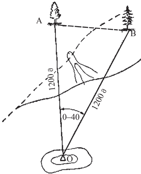
ტერიტორიაზე AB ხაზის გაზომვა OA=OB=1200 \text{ მ}
